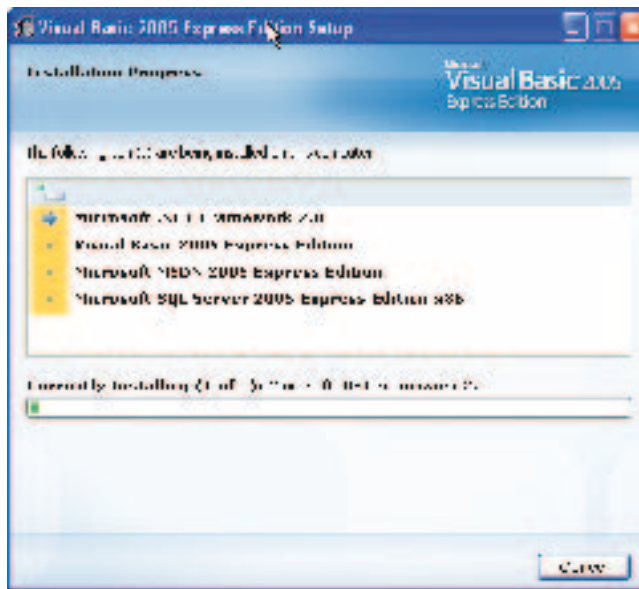
Figur 2-7 Installationsprocessen.
